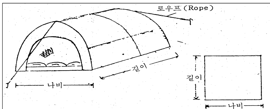
그림 1 - 반원통형텐트
